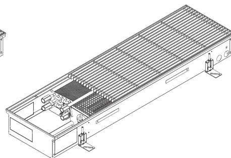
System 4-rurowy
