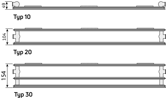
Widoki z góry
