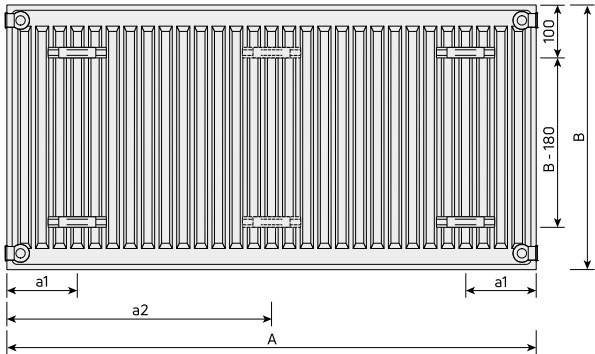
Widoki z tyłu (typy 20, 30)
